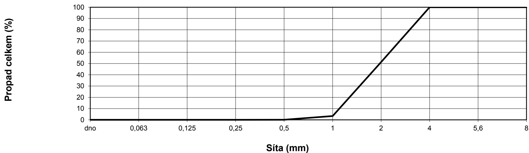
Křivka zrnitosti
