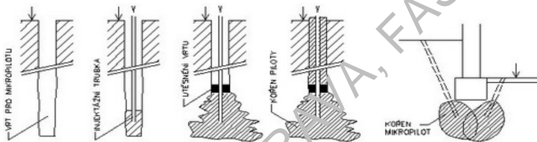
Mikropiloty a kořenové piloty
