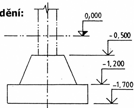
Základová patka
