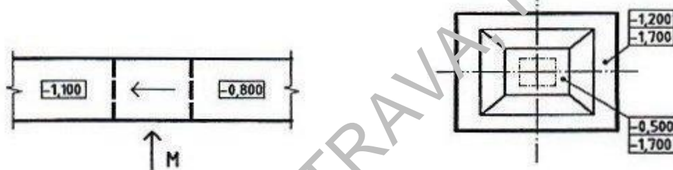
Základy zakreslování - případ c
