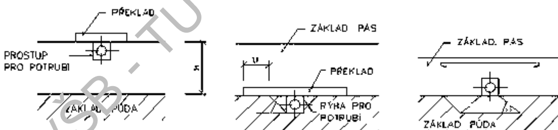
Konstrukční úpravy – prostupy v základech
