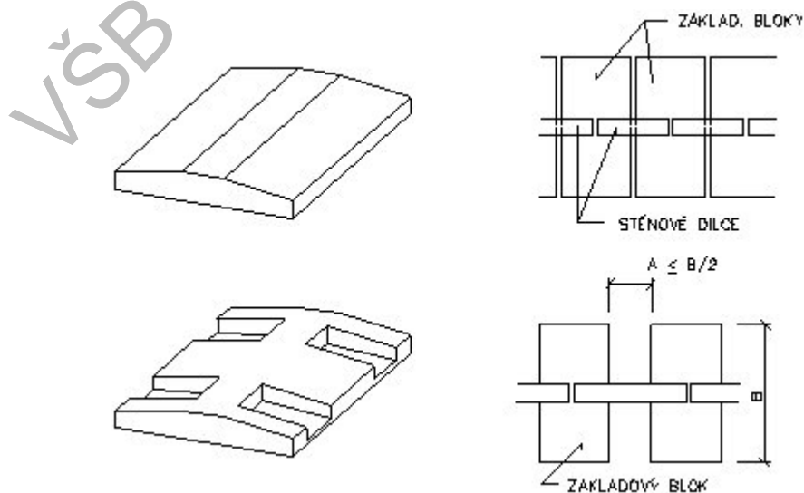
Základový pás - prefabrikovaný
