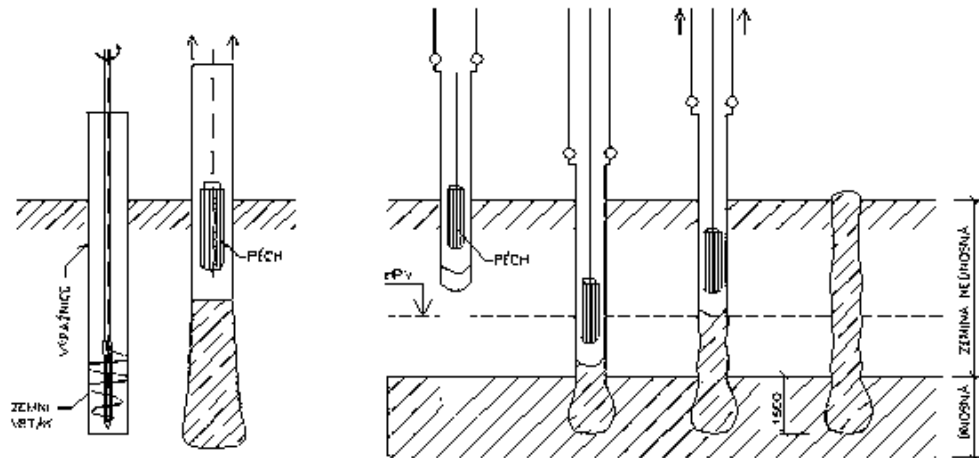
Železobetonové monolitické piloty - vrtané s odňatou výpažnicí
